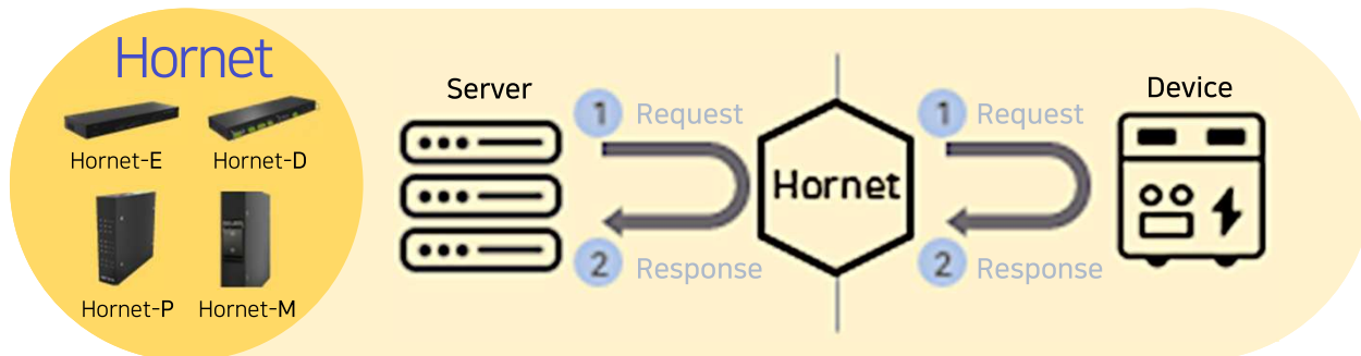
3-tier 방식 독립형 데이터 전송
